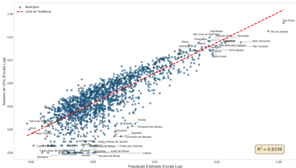
Figura 4 – Dispersão entre População Estimada e UHs Contratadas na Região Sudeste
